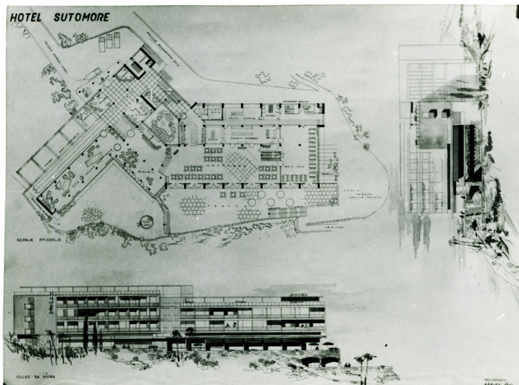
Hotel u Sutomoru, osnova, fasade (Fond Muzeja nauke i tehnike, poklon autora)
